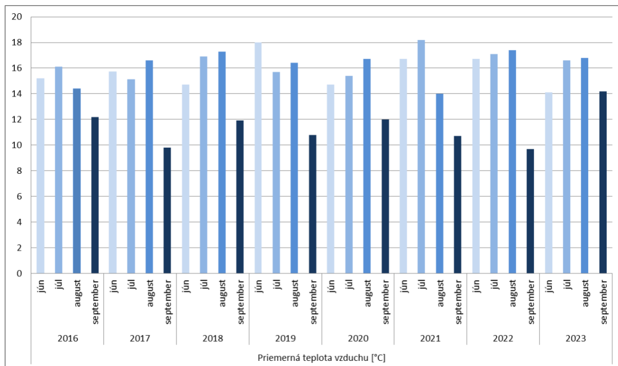
Obr. 2: Priemerná teplota vzduchu na VUK Palcmanová Maša (zdroj: SHMÚ)
